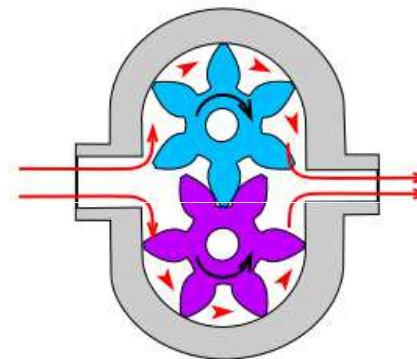
Pompa ad ingranaggi
