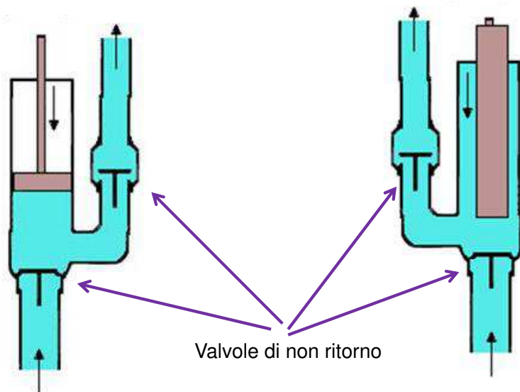
Pompa a stantuffo
