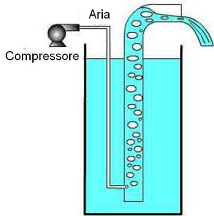
Pompa ad aria compressa
