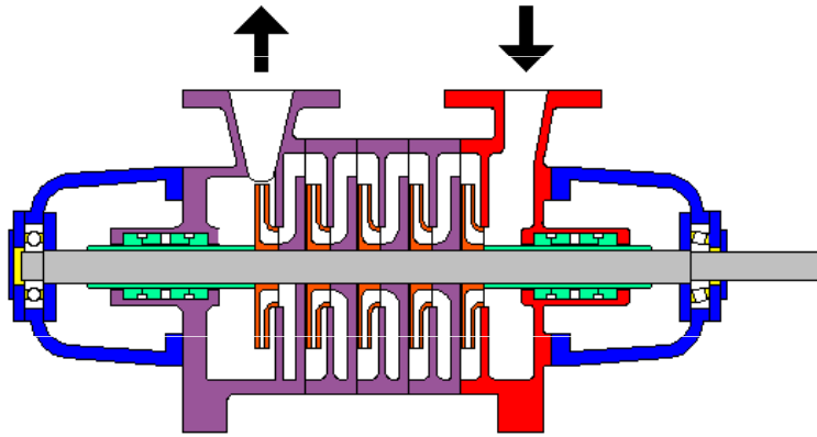
Pompa multistadio a 5 stadi
